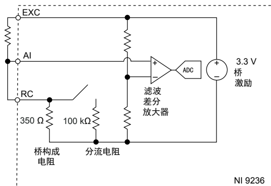
图 1. NI 9236 某通道的输入电路
