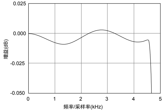
图 2. NI 9236 的典型通带响应
